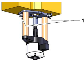
Рис. 93: Клапан линии охлаждения 2
