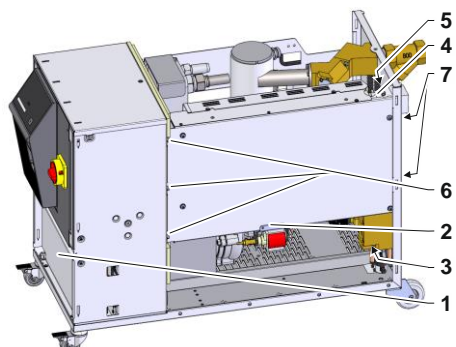
Рис. 95: Демонтаж нагревательного элемента, 32 кВт
