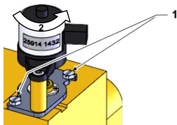
Рис. 92: Демонтаж клапана линии охлаждения 1
