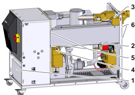
Рис. 94: Демонтаж нагревательного элемента, 16 кВт
