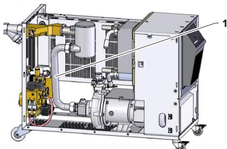
Рис. 91: Снять соединение с трубой
