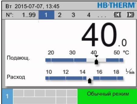
Рис. 40: Индивидуальное отключение
