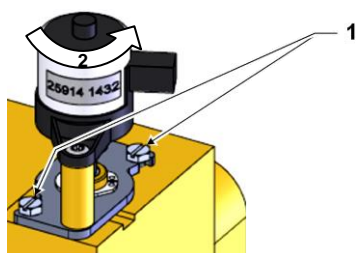
Фиг. 93: Демонтаж на охлаждащ вентил 1
