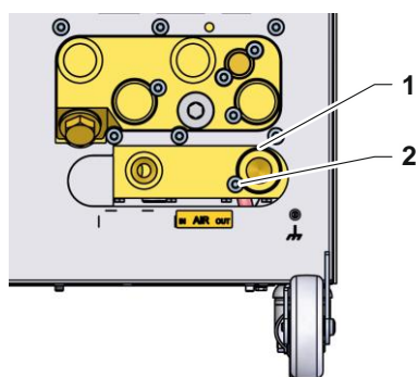
Фиг. 12: Изпразване изход със сгъстен въздух
