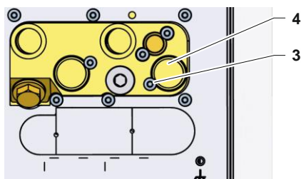
Фиг. 11: Отделна връзка за изходяща вода за охлаждане и от системата
