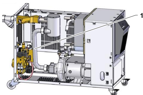
ábra 94: Csőcsatlakozás eltávolítása
