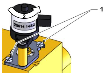
Ábra 95: Hűtőszelep 1 kiszerelese
