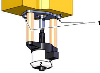
Ábra 96: Hűtőszelep 2
