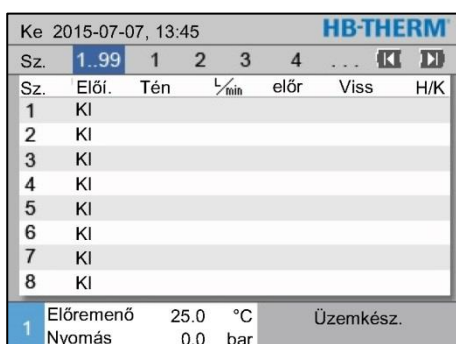
34. ábra: Táblázatos nézet
