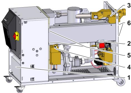
Fig. 90 : Retirer le chauffage 16 kW
