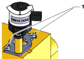
Fig. 89 : Dépose de la vanne de refroidissement 1
