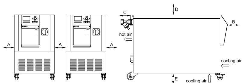
Fig. 3: Espace libre autour de l'appareil
