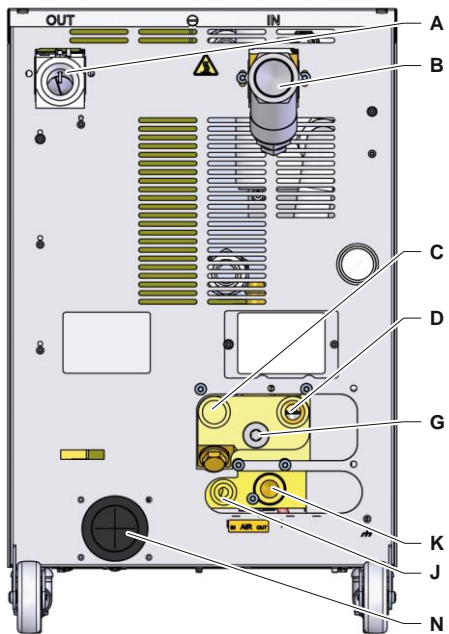
Fig. 5: Raccords
