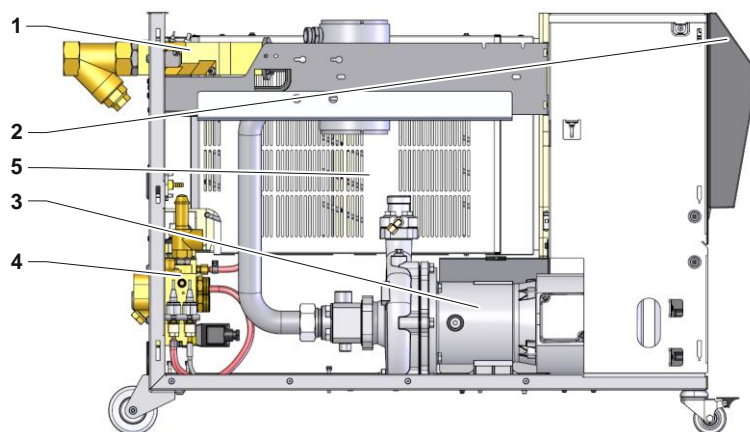
Fig. 4 : Vue d'ensemble
