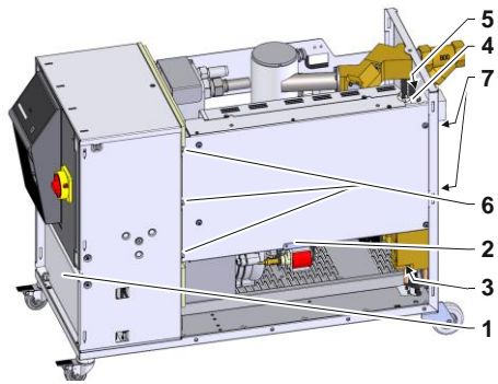
Fig. 91: Retirer le chauffage 32 kW
