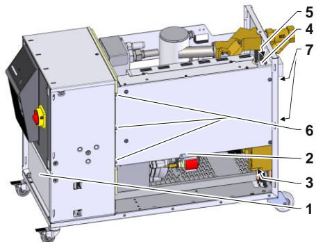
Fig. 93: Retirer le chauffage 32 kW
