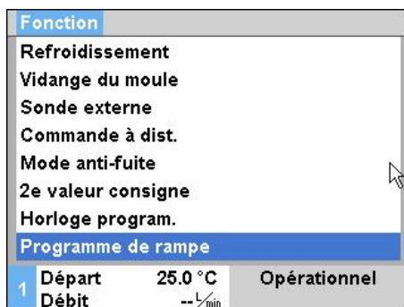
Fig. 66 : Programme de rampe
