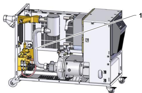
Fig. 90: Retrait du raccord de tuyau
