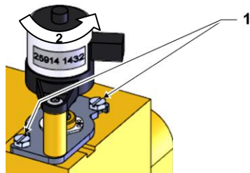
Fig. 91 : Dépose de la vanne de refroidissement 1
