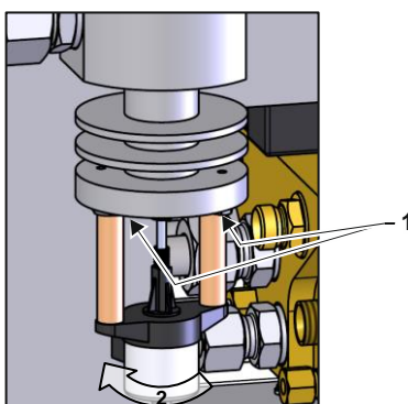
Рис. 94: Клапан линии охлаждения 2
