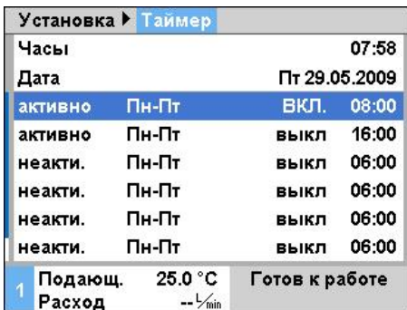
Рис. 66: Настройки таймера
