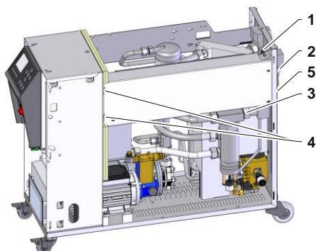
Рис. 92: Демонтаж термоэлемента
