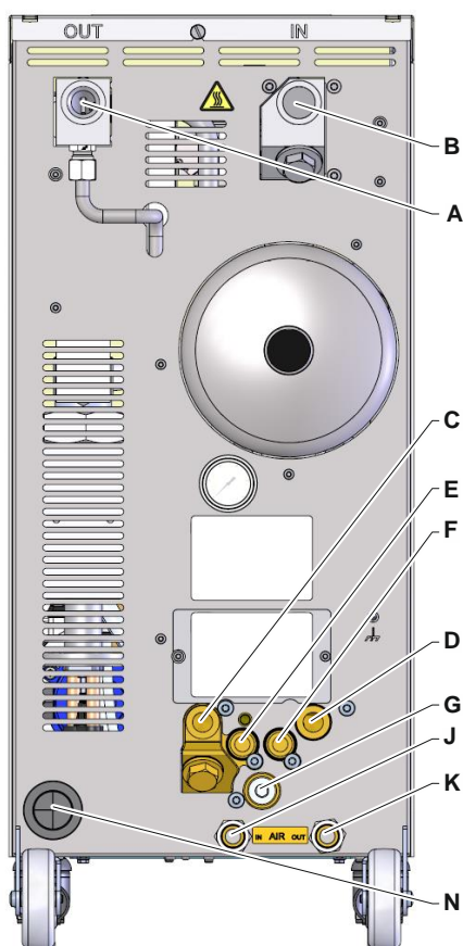
Рис. 5: Подключения
