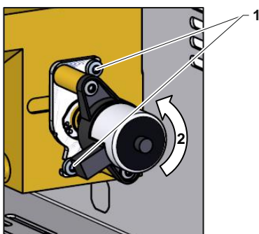
Afb. 94: Koelklep 1 demonteren
