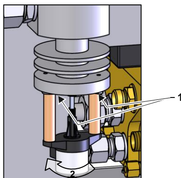
Afb. 95: Koelklep 2
