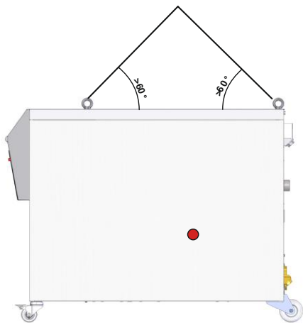
Afb. 7: Aanslagpunten
