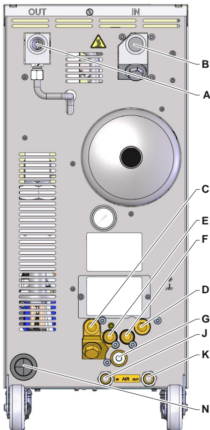
Afb. 5: Aansluitingen
