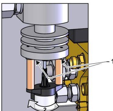
Sl. 97: Hladilni ventil 2
