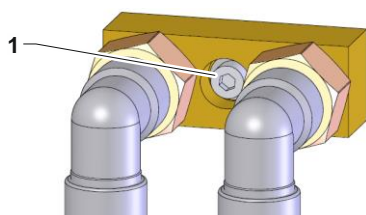
Sl. 12: Centralno pritrjevanje
