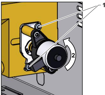
Afb. 96: Koelklep 1 demonteren
