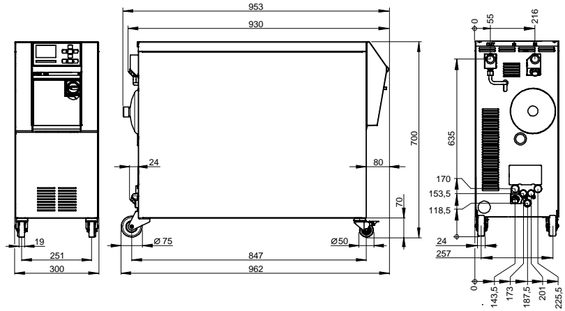
Abb. 2: Abmessungen
