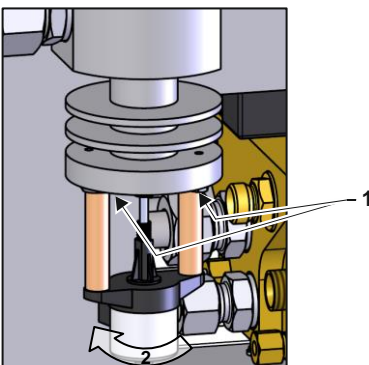
Abb. 97: Kühlventil 2
