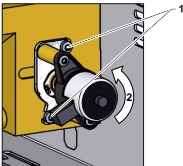
Abb. 96: Kühlventil 1 ausbauen
