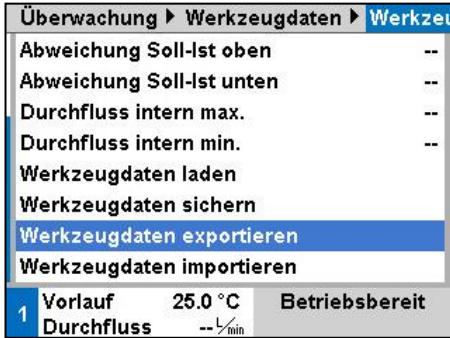
Abb. 86: Werkzeugdaten exportieren
