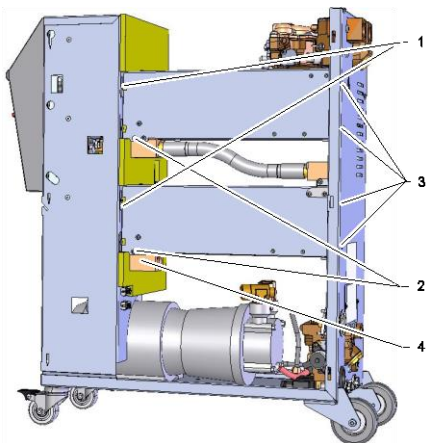
Фиг. 90: Демонтаж на подгряването
