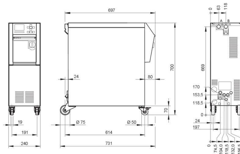
Рис. 2: Габариты
