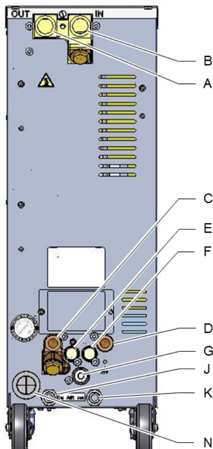
Рис. 5: Подключения
