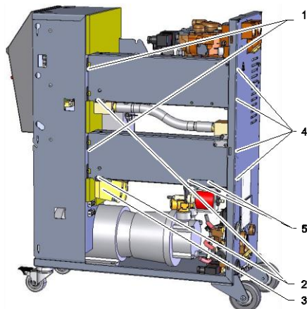
Рис. 95: Демонтаж термоэлемента
