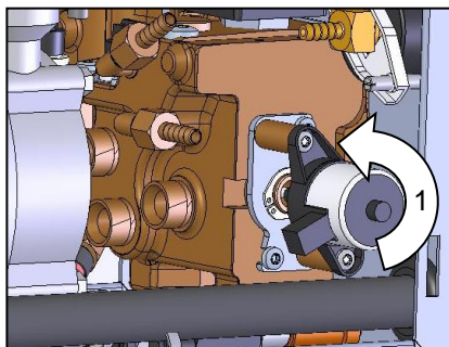
Sl. 93: demontaža hladilnega ventila 1
