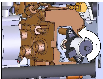
Obr. 93: Demontáž chladiaceho ventilu 1
