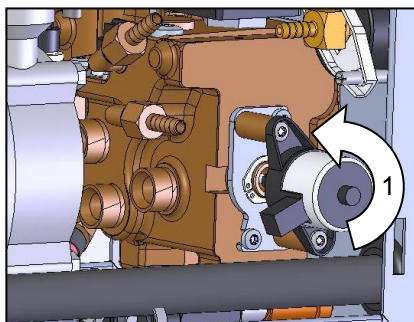
Afb. 93: Koelklep 1 demonteren
