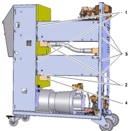
Fig. 92 : Déposer le chauffage
