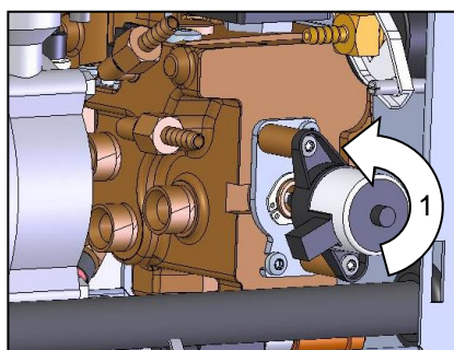
Fig. 93 : Dépose de la vanne de refroidissement 1
