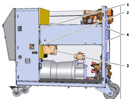
Sl. 90: demontaža gretja
