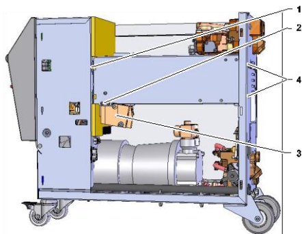
Рис. 90: Демонтаж термоэлемента
