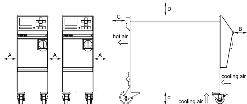
rys. 3: Wolne miejsce wokół urządzenia
