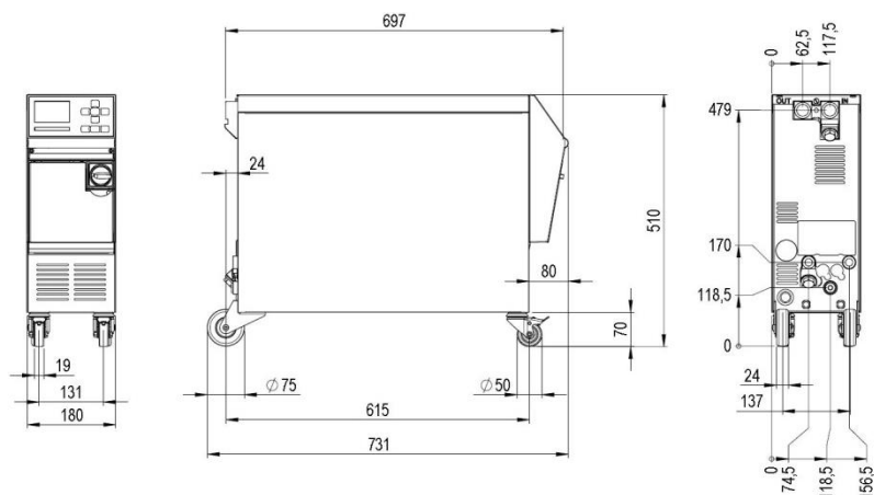
Rys. 2: Wymiary
