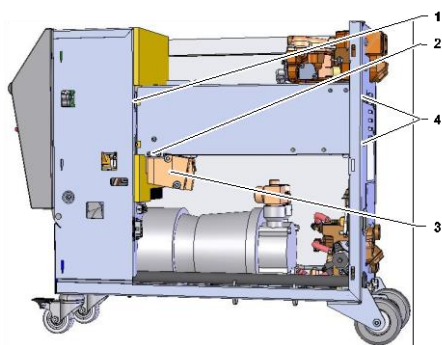
Fig. 90: Desmontar la calefacción
