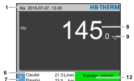
Fig. 20: Pantalla principal de aparato operado como módulo
