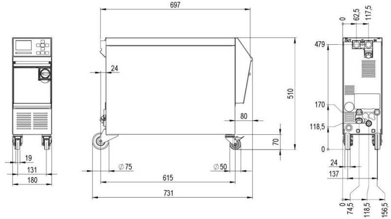
Fig. 2: Dimensiones
