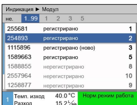
Фиг. 25: Индикация \ Действителни стойности
