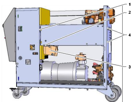
Bild 92: Demontera uppvärmningen
