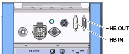
Sl. 16: Vmesniki Vario-5
