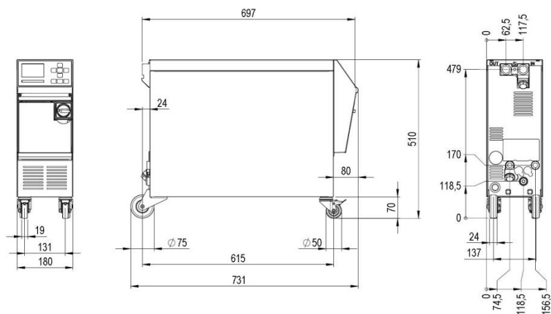
Obr. 2: Rozmery
