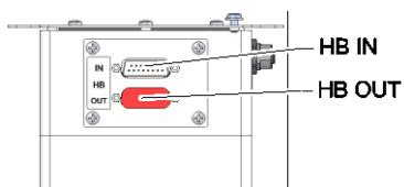
Obr. 15: Rozhrania Flow-5 Konštrukcia: Autonómny
