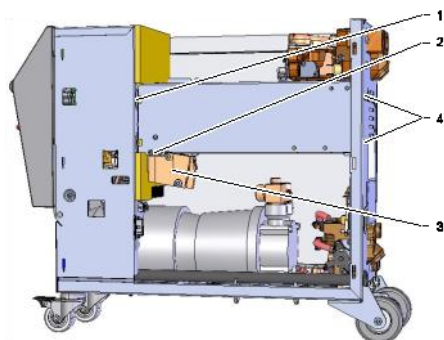
Obr. 92: Vymontovanie ohrevu
