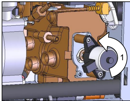
Afb. 93: Koelklep 1 demonteren
