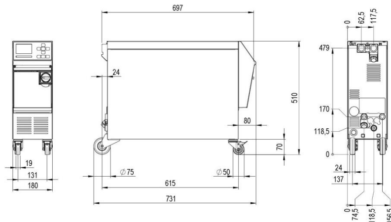
Fig. 2 : Dimensions
