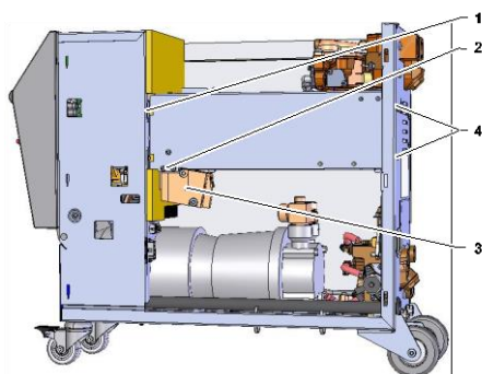
Fig. 92 : Déposer le chauffage
