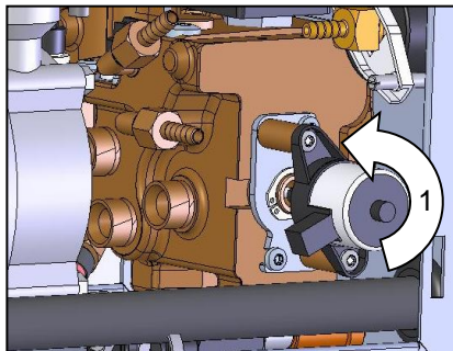
Kuva 93: Jäähdytysventtiilin 1 irrotus
