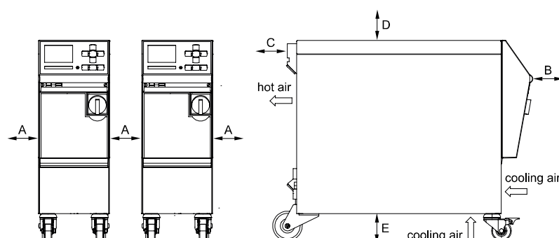
Фиг. 3: Свободно пространство около устройството
