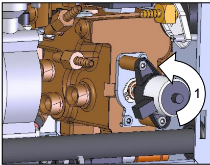
Abb. 95: Kühlventil 1 ausbauen
