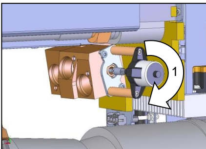
Abb. 96: Kühlventil 2
