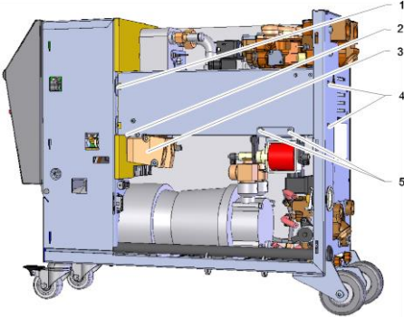
Abb. 94: Heizung ausbauen
