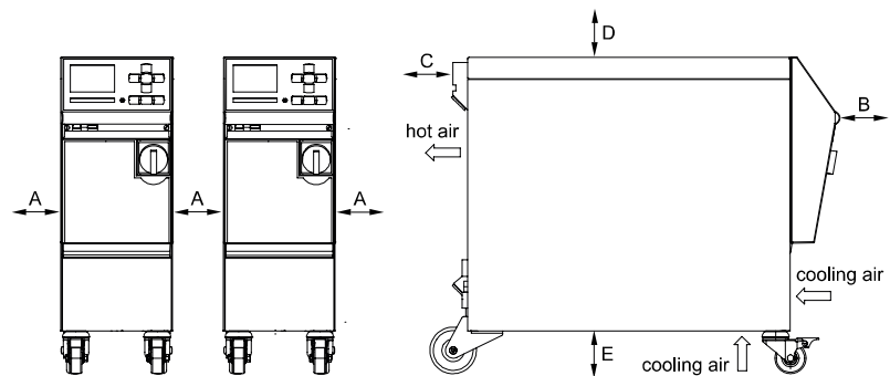
Abb. 3: Freiräume um das Gerät
