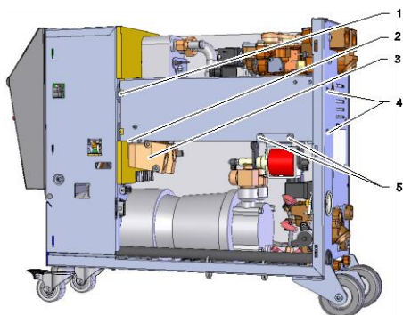
Obr. 96: Vymontovanie ohrevu
