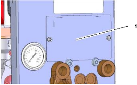
Obr. 99: Kryt ventilov
