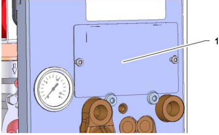
Afb. 99: Afdekking kleppen
