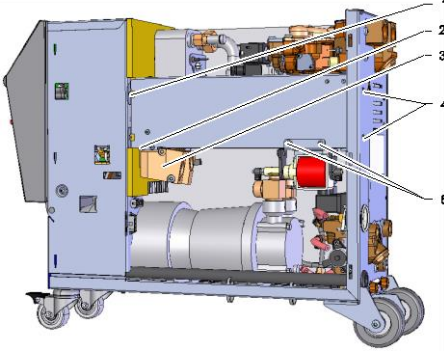
Afb. 96: Verwarming demonteren
