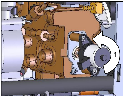
Afb. 97: Koelklep 1 demonteren
