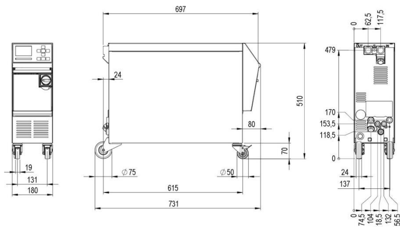
Fig. 2 : Dimensions
