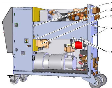
Fig. 96 : Déposer le chauffage
