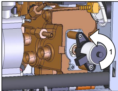
Abb. 97: Kühlventil 1 ausbauen
