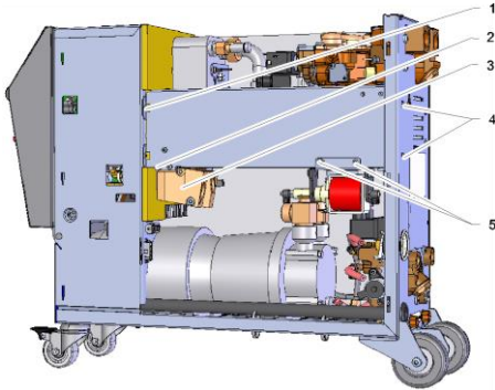
Abb. 96: Heizung ausbauen
