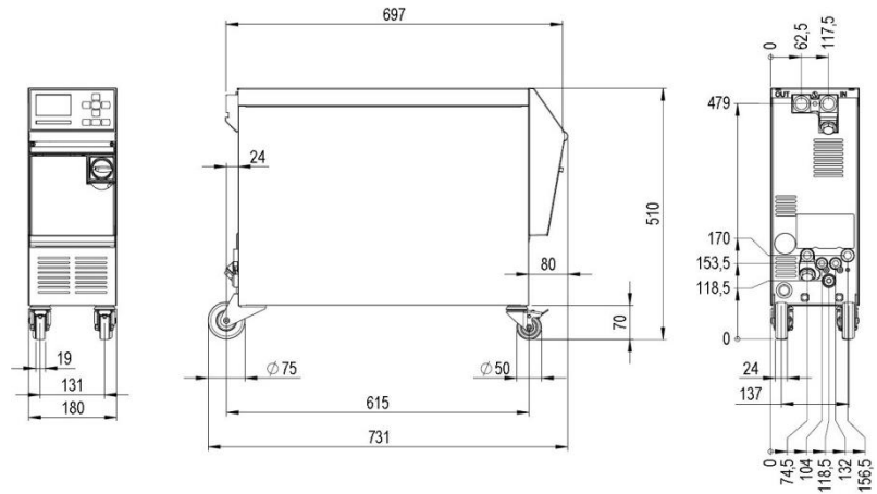
Abb. 2: Abmessungen
