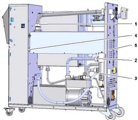
Рис. 73: Демонтаж термоэлемента
