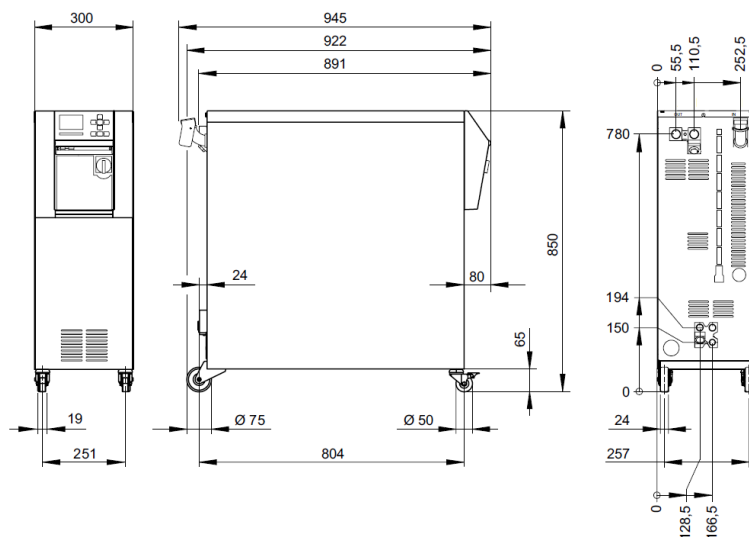
Рис. 2: Габариты
