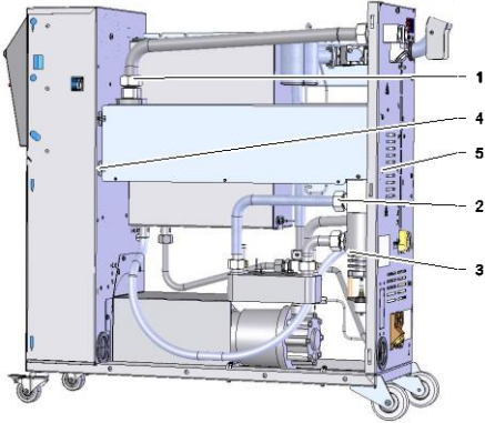
Afb. 73: Verwarming demonteren
