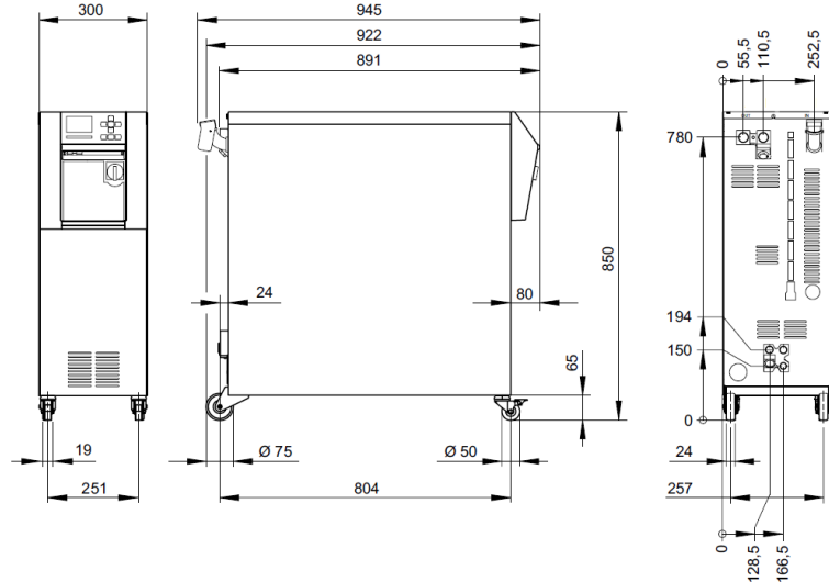
Afb. 2: Afmetingen
