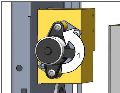
Afb. 74: Koelklep 1 demonteren
