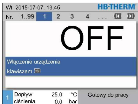
Rys. 31: Ekran podstawowy
