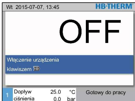
Rys. 30: Ekran podstawowy
