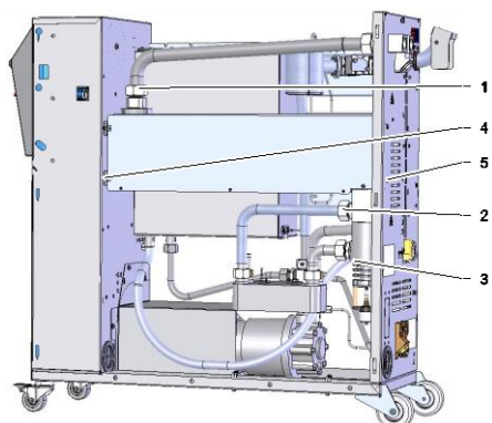
Rys. 75: Wymontować grzałkę
