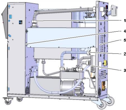
Abb. 75: Heizung ausbauen
