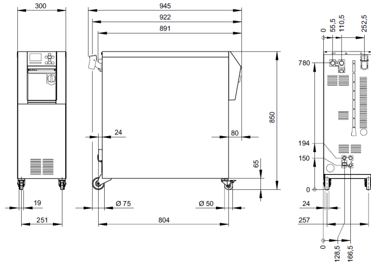
Abb. 2: Abmessungen
