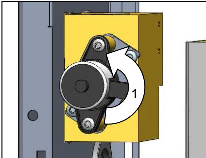
III. 76: Afmonter køleventil 1
