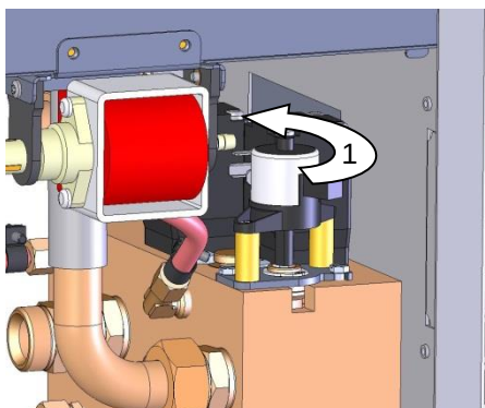
Sl. 77: demontaža hladilnega ventila 1
