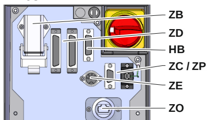
Sl. 12: Vmesniki samostojne naprave
