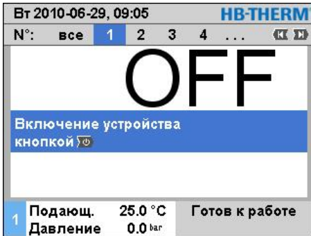
Рис. 29: Главное окно
