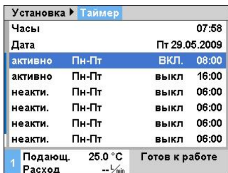
Рис. 54: Настройки таймера
