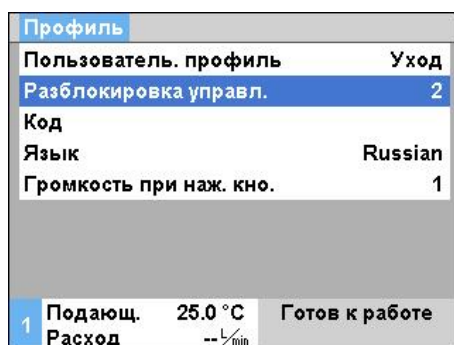
Рис. 49: Разблокирование управления
