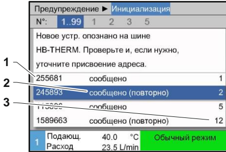
Рис. 24: Инициализация
