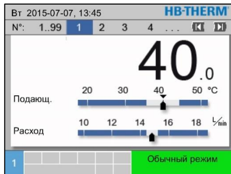
Рис. 39: Индивидуальное отключение
