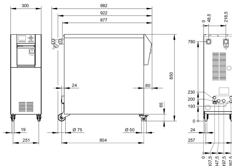
Рис. 2: Габариты
