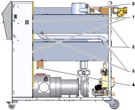
Фиг. 80: Демонтаж на подгряването
