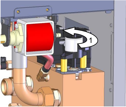
Fig. 79 : Dépose de la vanne de refroidissement 1
