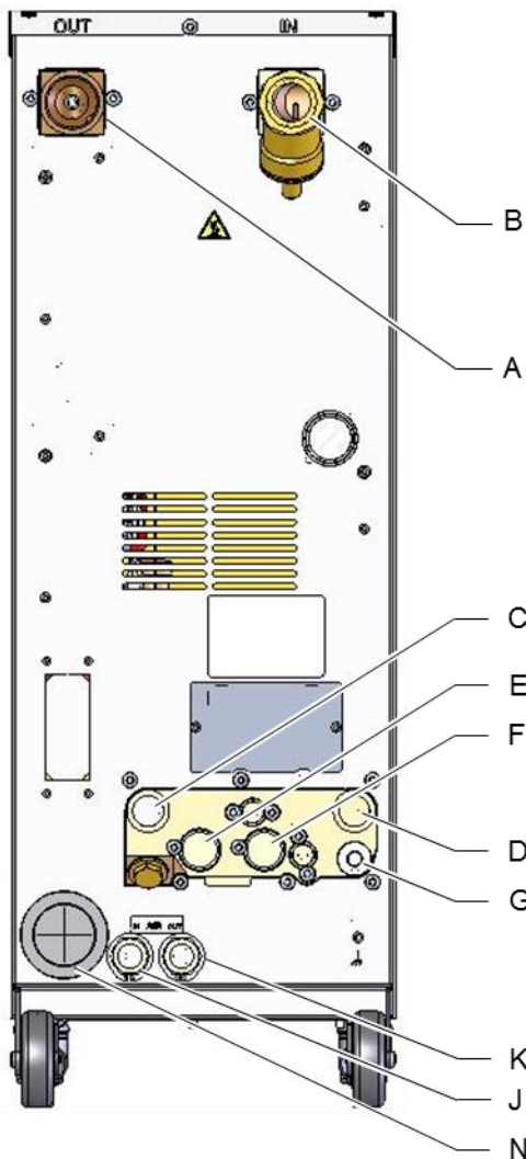
Fig. 5 : Raccords
