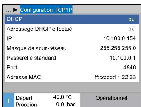
Fig. 41: Paramètres réseau
