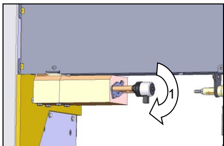
Фиг. 80: Охлаждащ вентил 2
