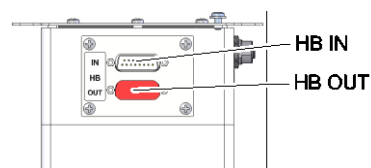
Фиг. 16: Интерфейси Flow-5 Модел: Автономен
