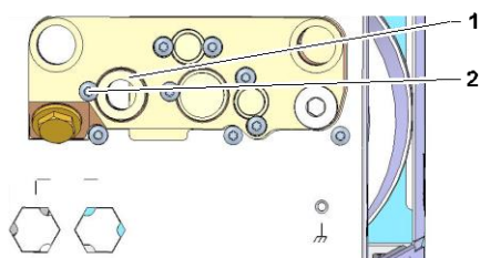
Фиг. 10: Отделна връзка за постъпваща вода за охлаждане и за системата
