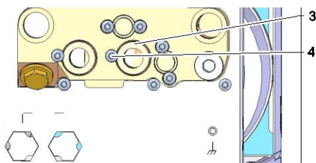
Фиг. 11: Отделна връзка за изходяща вода за охлаждане и от системата
