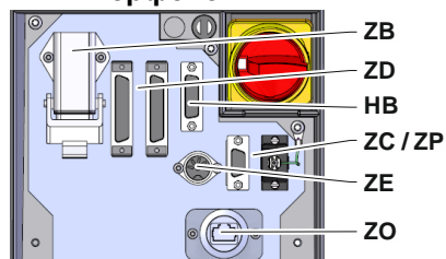
Фиг. 12: Интерфейси отделно устройство
