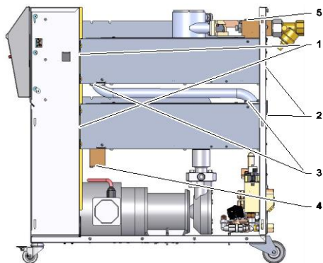
Фиг. 82: Демонтаж на подгряването
