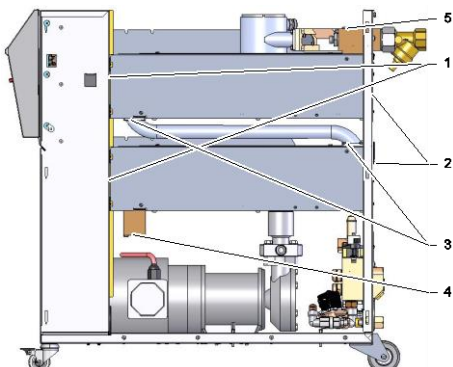
Рис. 77: Демонтаж термоэлемента
