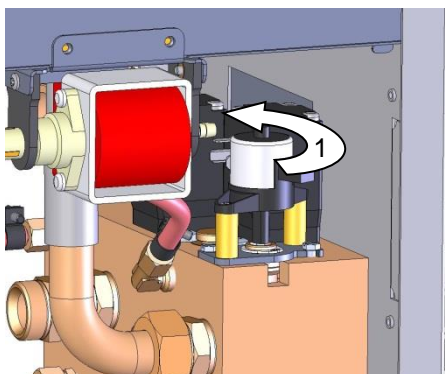
Fig. 76 : Dépose de la vanne de refroidissement 1
