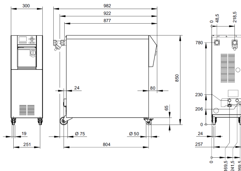
Fig. 2 : Dimensions
