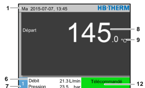
Fig. 21: Premier niveau d'affichage Appareil piloté comme module
