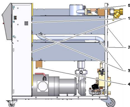
Fig. 77 : Déposer le chauffage
