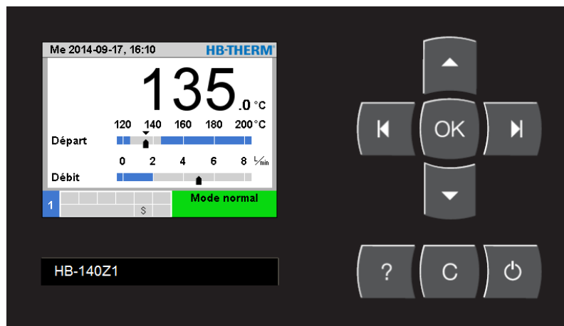
Fig. 17 : clavier et affichage
