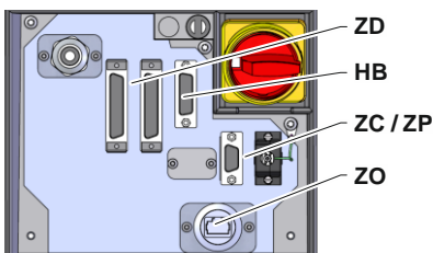
Abb. 12: Schnittstellen Panel-5
