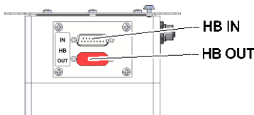
Abb. 14: Schnittstellen Flow-5 Bauart: Autonom
