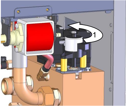
Abb. 76: Kühlventil 1 ausbauen
