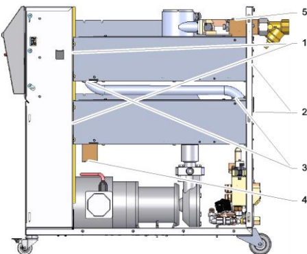
Abb. 77: Heizung ausbauen
