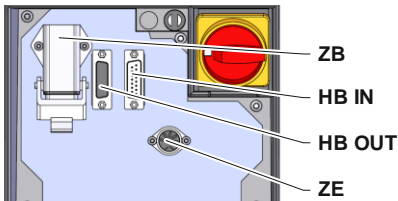
Abb. 11: Schnittstellen Modulgerät
