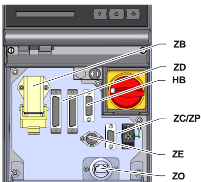
Abb. 16: Schnittstellen Einzelgerät
