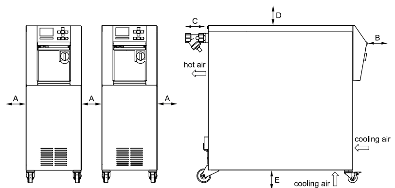
Abb. 3: Freiräume um das Gerät
