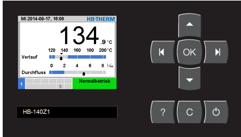
Abb. 17: Tastatur und Anzeige
