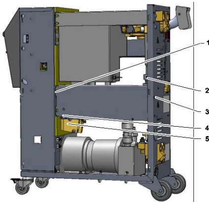
Bild 74: Demontera uppvärmningen
