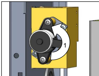
Bild 75: Demontera kylventil 1
