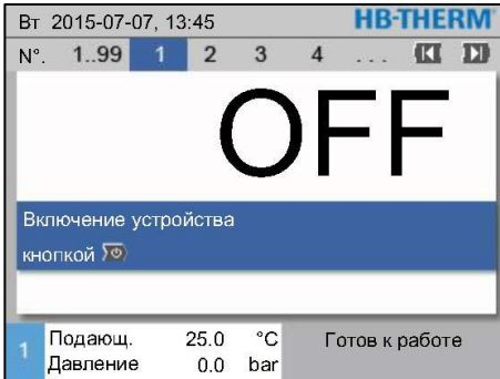
Рис. 29: Главное окно
