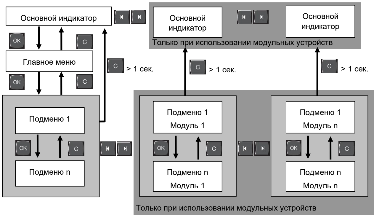
Рис. 22: Структура управления
