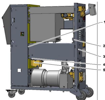
Рис. 74: Демонтаж термоэлемента
