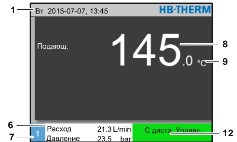
Рис. 21: Основное поле индикации, управление устройством как модулем
