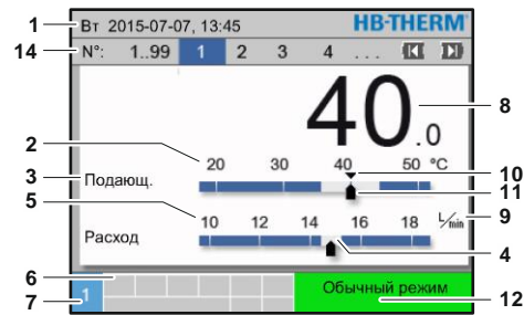
Рис. 19: Основное поле индикации, график
