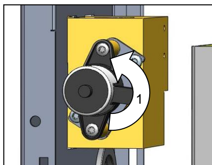
Рис. 75: Демонтаж клапана линии охлаждения 1
