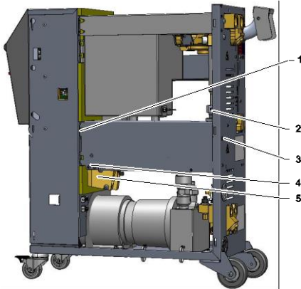
Afb. 74: Verwarming demonteren
