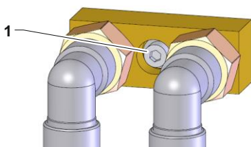
Fig. 10: Fixation centrale
