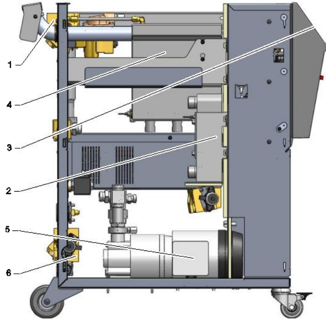
Fig. 4 : Vue d'ensemble
