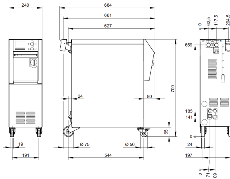
Fig. 2 : Dimensions
