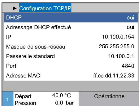
Fig. 38: Paramètres réseau
